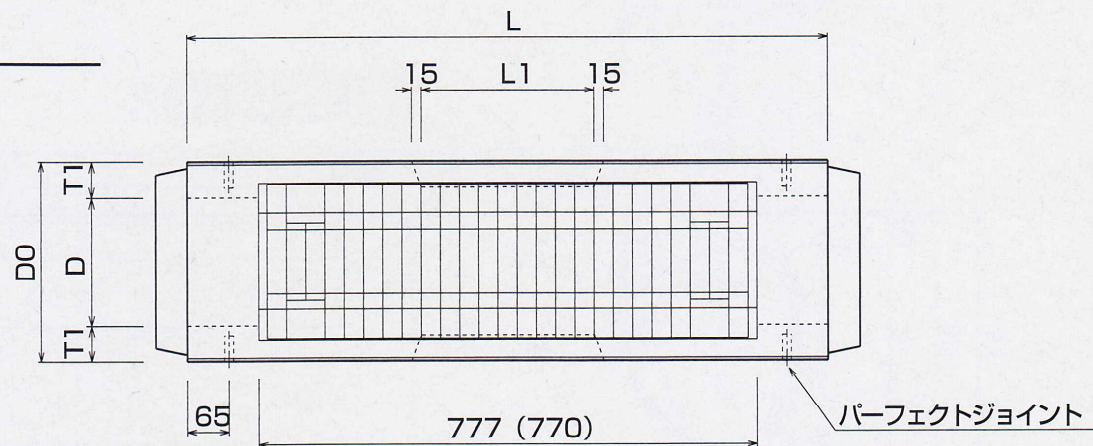
平面図
