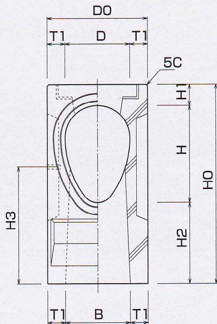
寸法表
